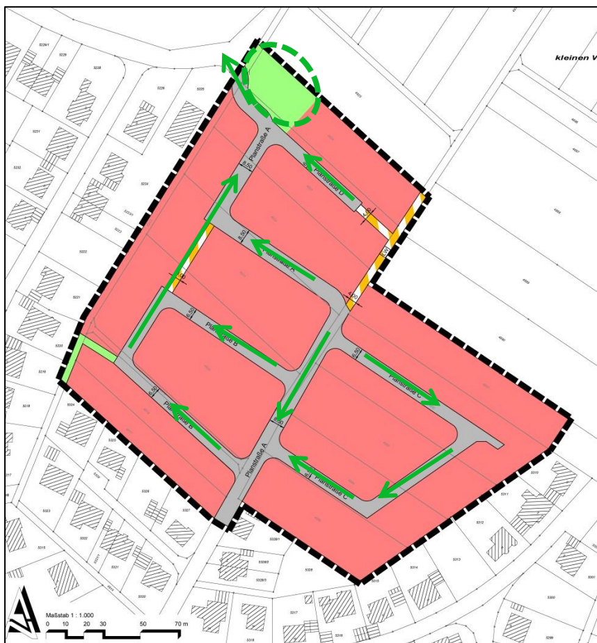
Abb. 10: Entwässerungssystem
